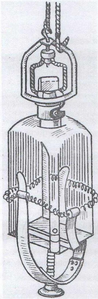
Рис. 1 . Батометр
